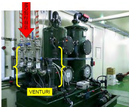
尾气处理器
